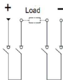
Type C wiring mode
