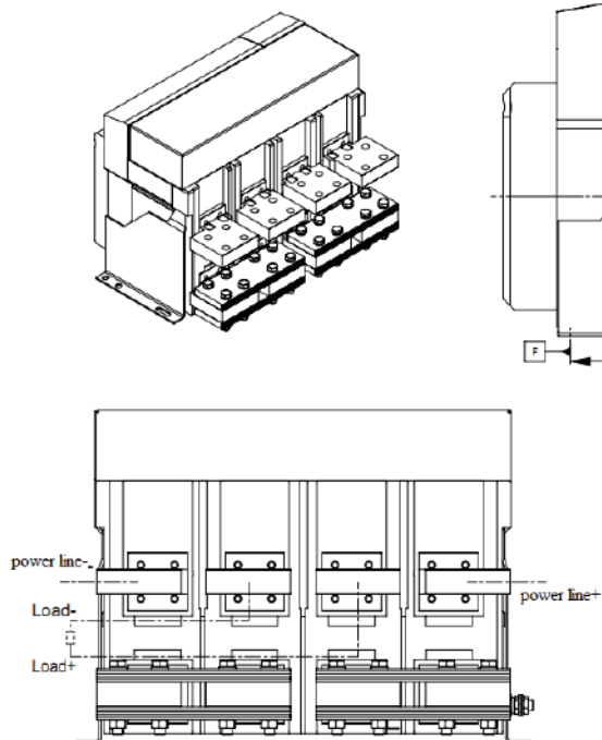
Dimensions
