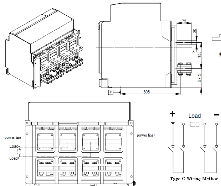
Dimensions
