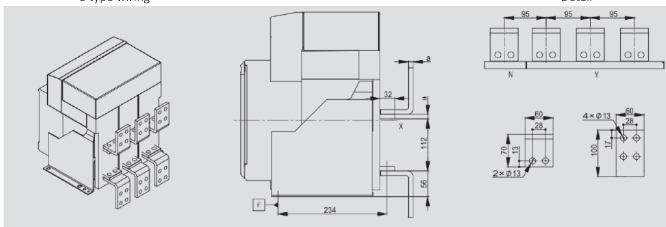
L-type wiring
