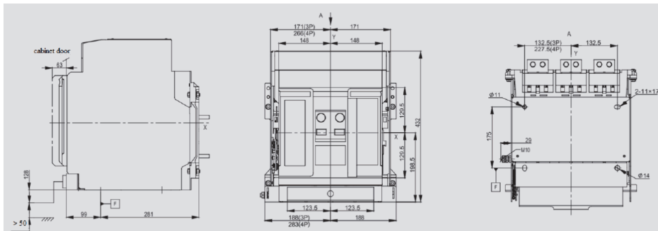
Horizontal Wiring
