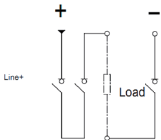
Type B wiring mode
