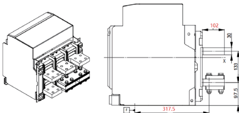
Dimensions
