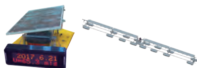
Floating PV tracking mounting system floSolar® 不銹鋼水面漂浮追日太陽能發電系統 floPV® 高密度聚乙烯水面漂浮太陽能發電系統
