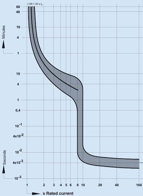
G characteristic I_n = 0,3 - 10 \text{ A} UL
